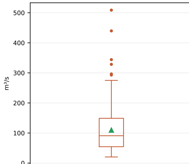
Q observado
