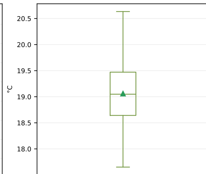
Tmedia estimada
