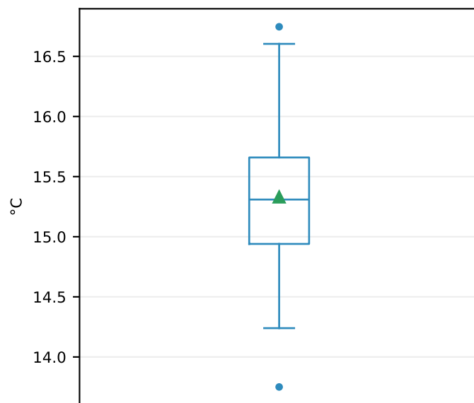
Media mensual Tmin
