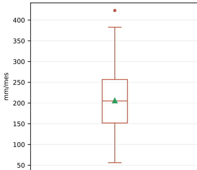
P IMERG
