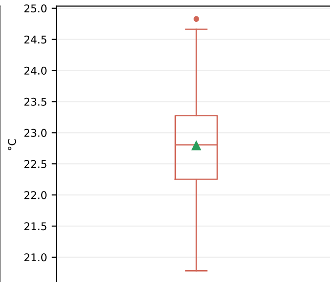
Media mensual Tmax
