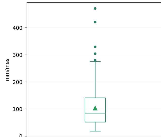
R escorrentía
